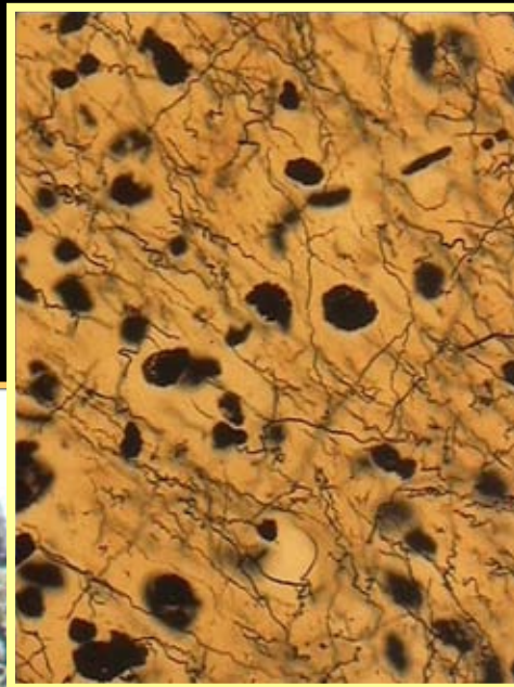
Cerebro. Células piramidales. Impregnación argéntica
