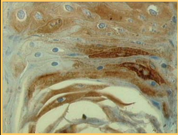
Lengua. Cara dorsal. Citoqueratinas 5/6. (Dr Rugani).
